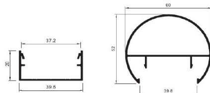
AD-1774 Anclaje telescópico pasamanos red 60
